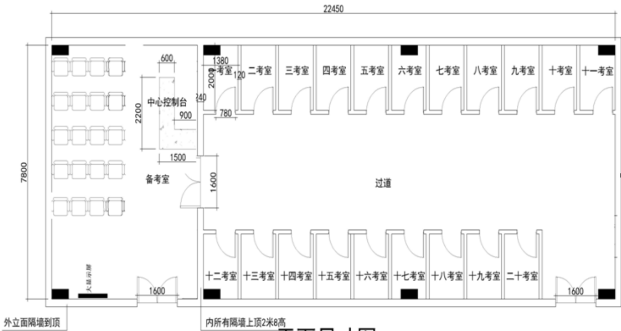
平面尺寸图
